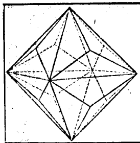
c. Triakis octahedron.
