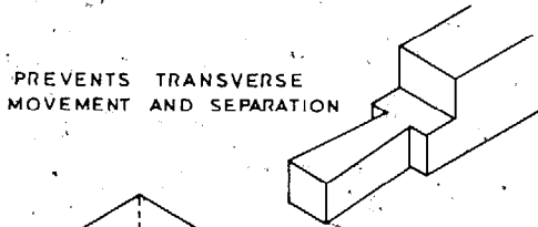
MORTISE & TENON
