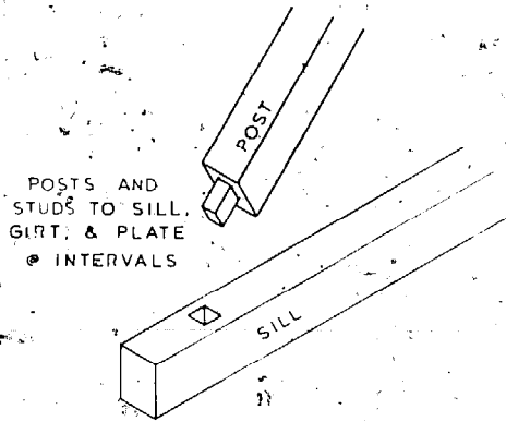
MORTISE & TENON
