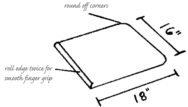
A.35: Sheet Metal Slider
