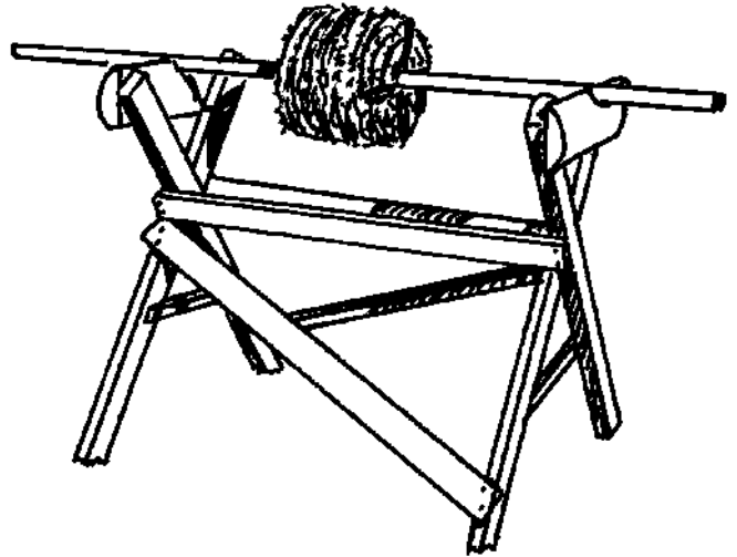
A.37: Buck stand barbed wire holder
