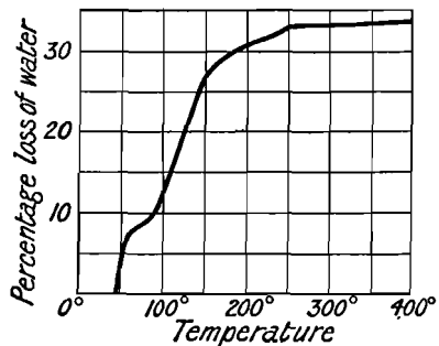
FIG. 28.—Dehydration Curve of Ulexite, \text{Na}_2\text{O} \cdot 2\text{CaO} \cdot 5\text{B}_2\text{O}_3 \cdot 16\text{H}_2\text{O} .
