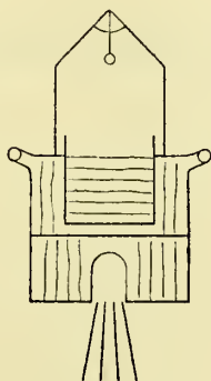
Appareil à sublimation.
